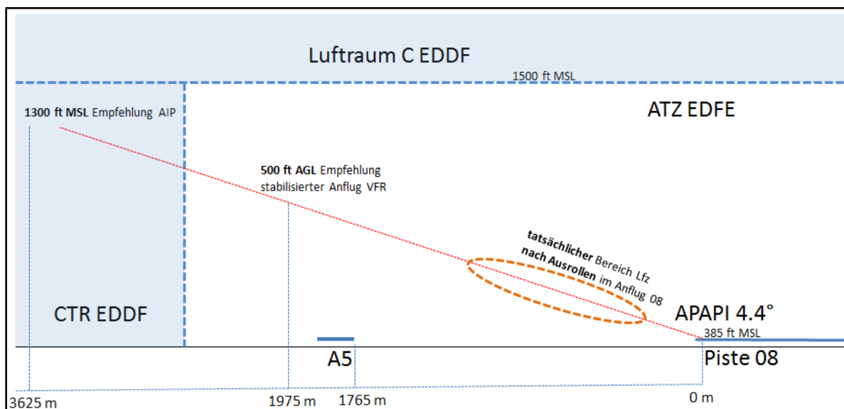
Abb. 23: Überblick Anflug auf die Piste 08 mit APAPI-Gleitwinkel
