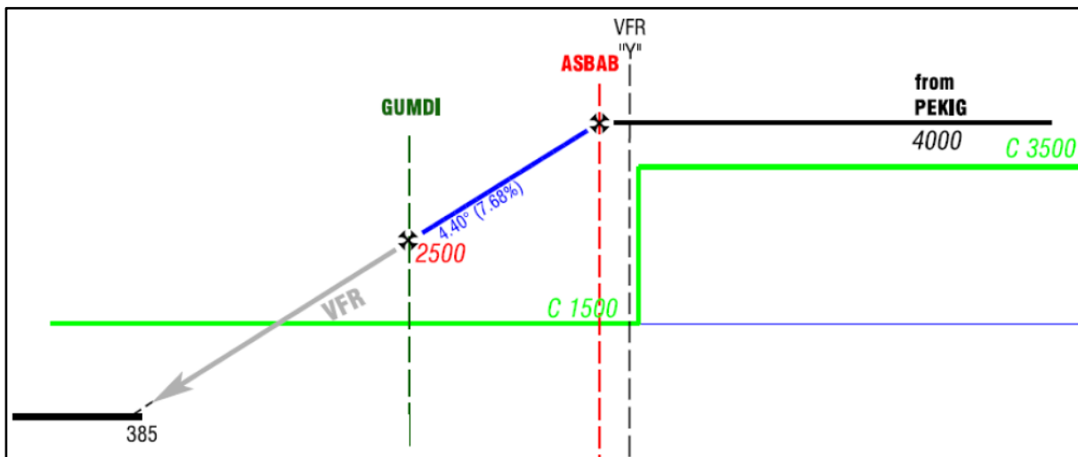
Abb. 18: Anflugprofil RWY26
